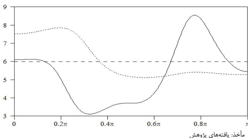
نمودار ۵. رابطه تورم (منحنی ممتد) و پایه پولی (منحنی نقطه‌چین) در فرکانس‌های بالا و پایین
