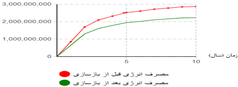
شکل ۴: نمودار مصرف انرژی قبل از بازسازی و بعد از بازسازی
