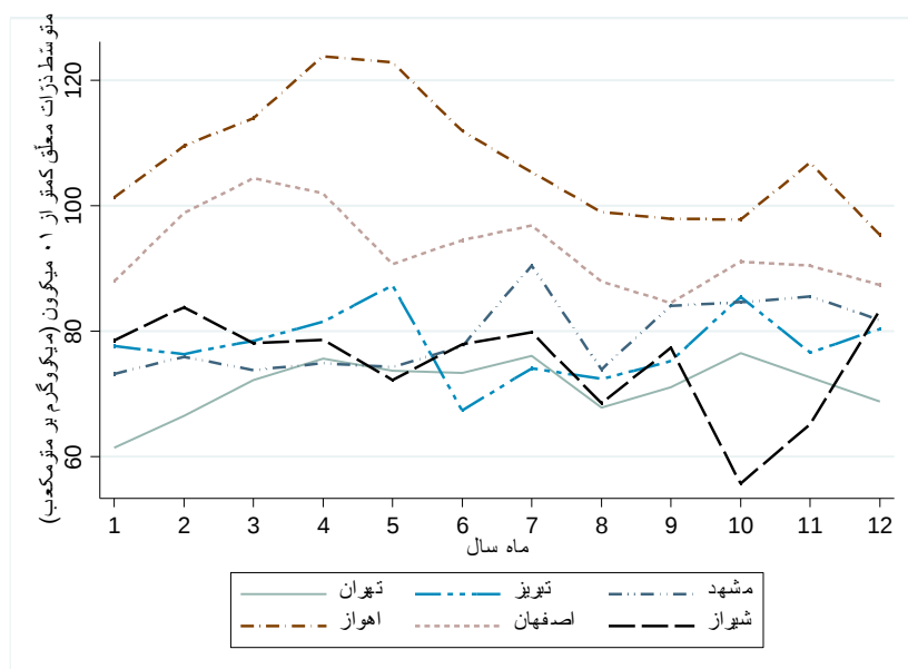
نمودار ۲. الگوی سالیانه تغییرات میزان ذرات کمتر از ۱۰ میکرون در طول سال در شهرهای مختلف
