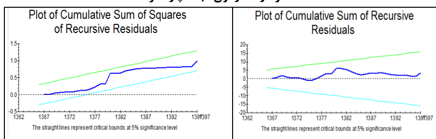
نمودار ۱. آزمون ثبات پارامترها
